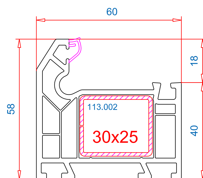
Рама 58 mm Арт.-№: 101.315 замена 101.010
