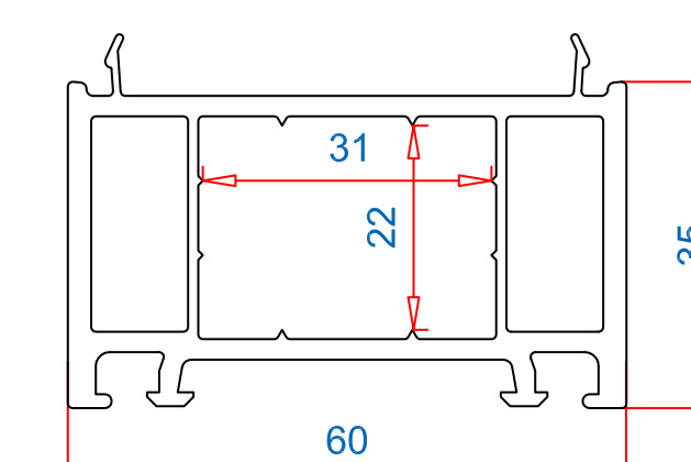
Расширитель 35 mm Арт.-№: 114.064 Усилитель: 30x20
