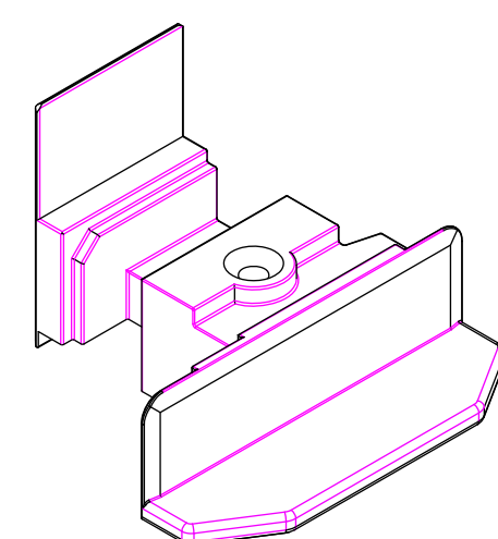
Заглушка штульпа Арт.-№: 109.257
