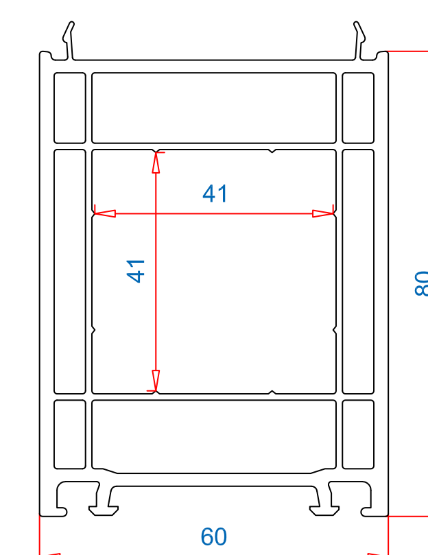
Расширитель 80 mm Арт.-№: 114.065 Усилитель: 40x40
