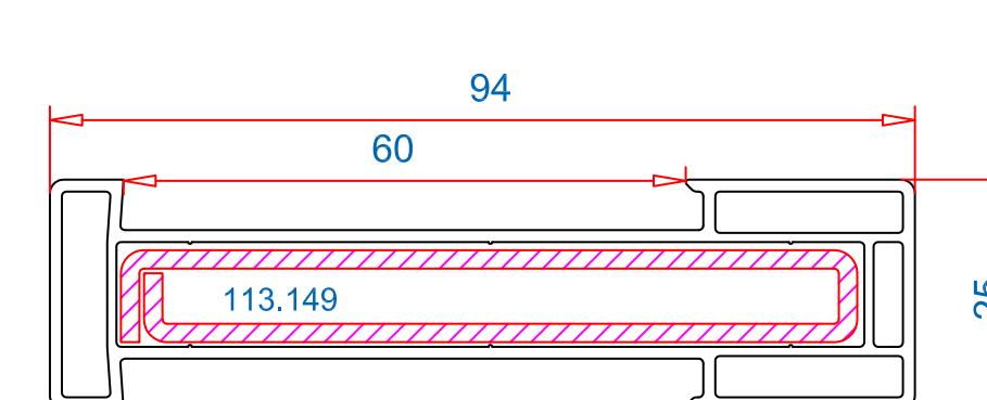
Соединитель 25mm Арт.-№: 116.044.2 Усилитель 113.149.2
