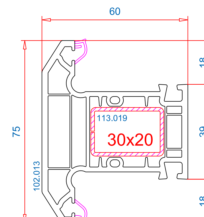
Импост 75 mm Арт.-№: 102.013 Усилитель: 113.019 Уплотнитель: 112.373
