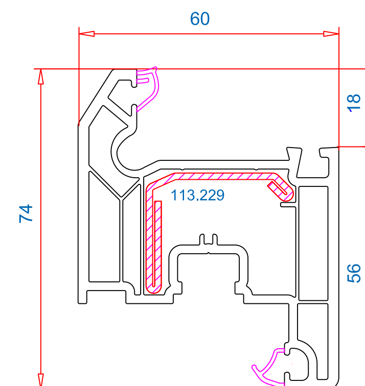
Створка 74 mm Арт.-№: 103.379 замена 103.011
