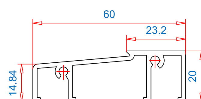
Алюминиевый порог 60x20 Арт.-№: 104.002
