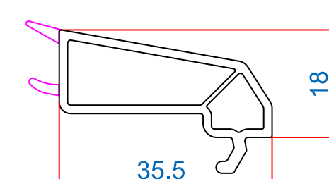
Штапик 35.5mm Арт.-№: 107.284 для стекла 4mm
