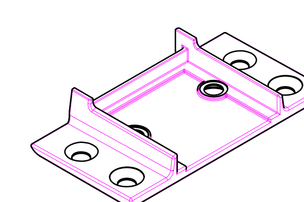
Соединитель импоста Арт.-№: 106.318.1 для 102.013
