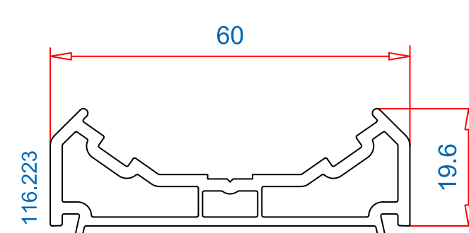
Соединительный профиль 60 mm Арт.-№: 116.223 для 116.225
