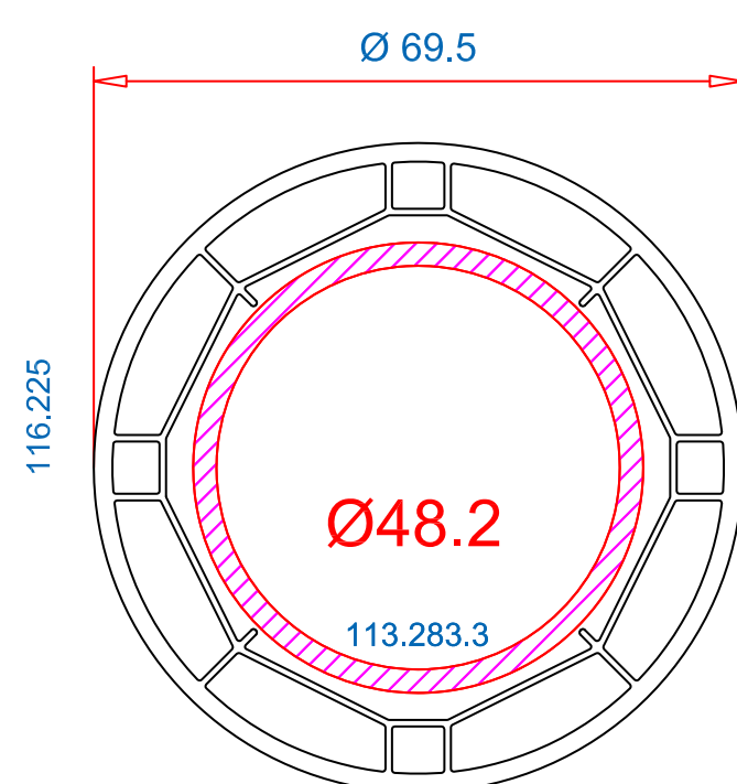
Соединитель круглый 70mm Арт.-№: 116.225 Усилитель: 113.283.3
