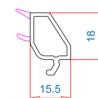
Штапик 15.5mm Арт.-№: 107.140 для с/п 24mm
