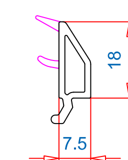
Штапик 7.5mm Арт.-№: 107.141 для с/п 32mm
