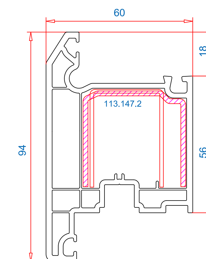
Створка нсв.н.о 94mm Арт.-№: 103.397 Усилитель: 113.147.2
