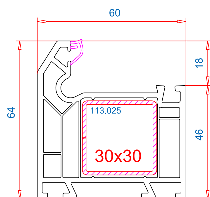
Рама 64 mm Арт.-№: 101.020 Усилитель: 113.025 Уплотнитель: 112.373
