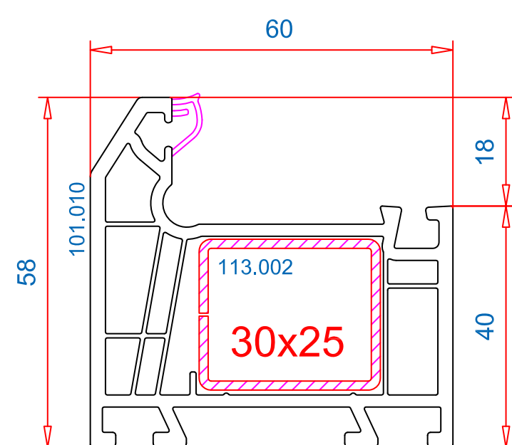
Рама 58 mm Арт.-№: 101.010 Усилитель: 113.002 Уплотнитель: 112.373
