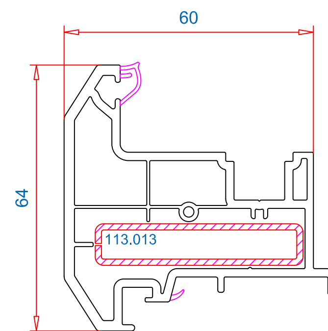
Штульп 64mm Арт.-№: 102.329 Усилитель: 113.013
