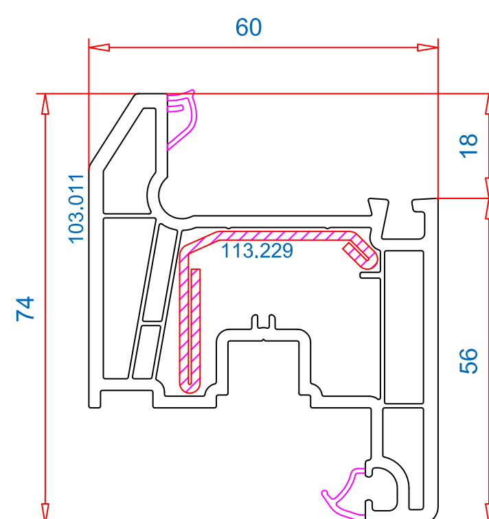
Створка 74 mm Арт.-№: 103.011 Усилитель: 113.229 Уплотнитель: 112.373/112.334
