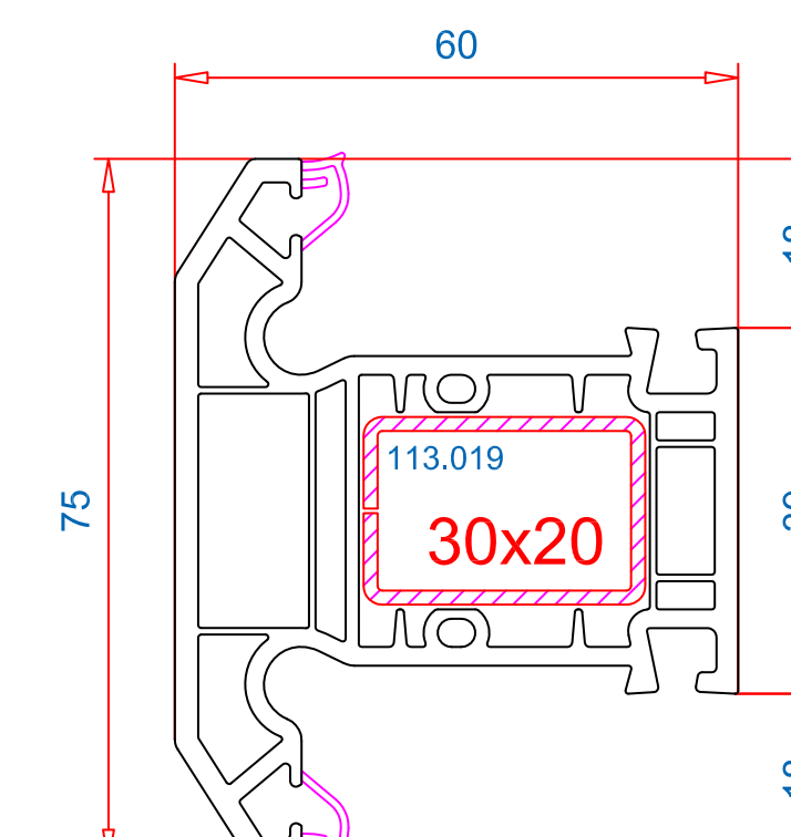
Импост 75 mm Арт.-№: 102.345 замена 102.013
